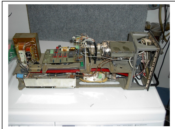
Baugruppen aus FUBA-Oszillator-Vervielfacherbaugruppen der alten 60-Ohm TV-Umsetzertechnik
